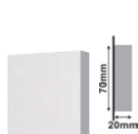
Roseta 175 | Rosette | Roseta 70 x 70 x 20mm Cód. | Code - 24347
