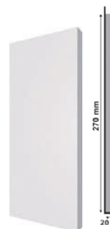
Sócalo 182 Plinth Block | Zócalin 110 x 270 x 20mm Cód. | Code - 24342
